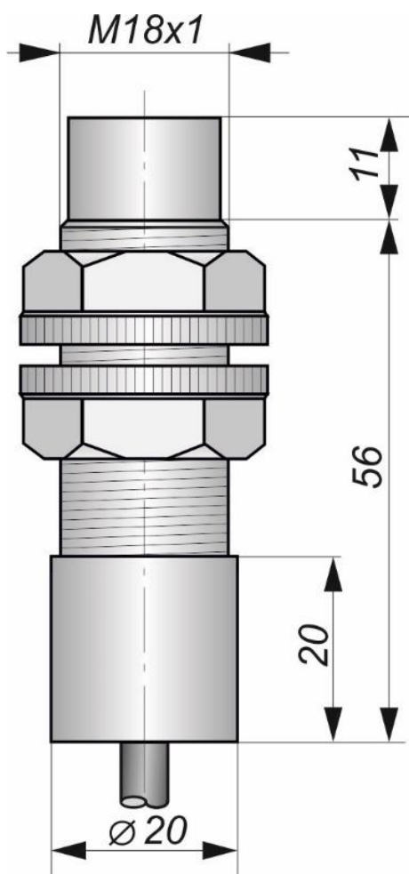
Габаритный чертеж
